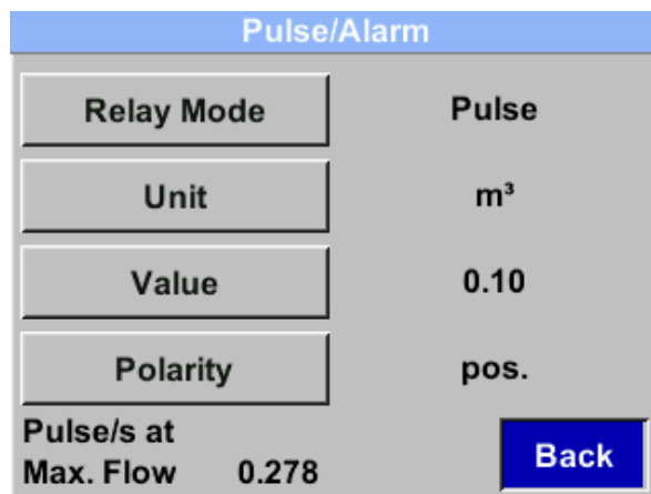
Figura 24: Configurazione dell'uscita a separazione galvanica (esempio)
