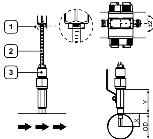
Figura 5: Allineamento del sensore (esempio)
