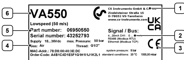
Figura 2: Targhetta (esempio)
