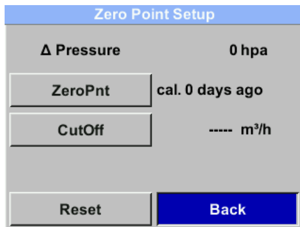
Figura 27: Esecuzione della regolazione del punto zero (esempio)
