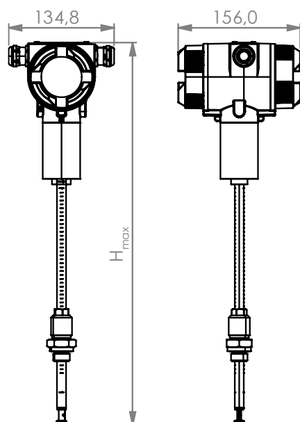
Figura 32: dimensioni
