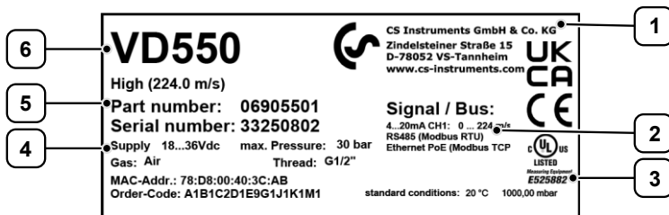
Figura 2: Targhetta (esempio)
