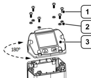
Figure 6: Tourner le couvercle du boîtier (exemple)
