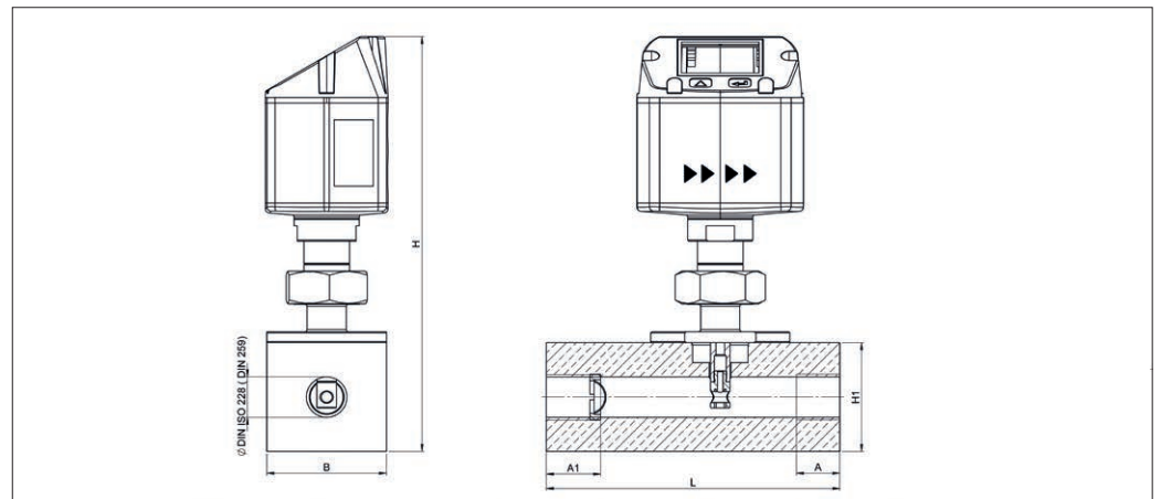
Mätområden flöde VA 521 (max-version 185 m/s) för tryckluft (ISO 1217:1000 mbar, 20 °C) Mätområden för andra gastyper, se sid. 118 till 121
