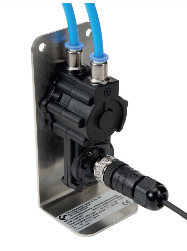
Typisk användningsplats för differenstryckmätning i kombination med två PE-slangar före och efter filterelementen.
