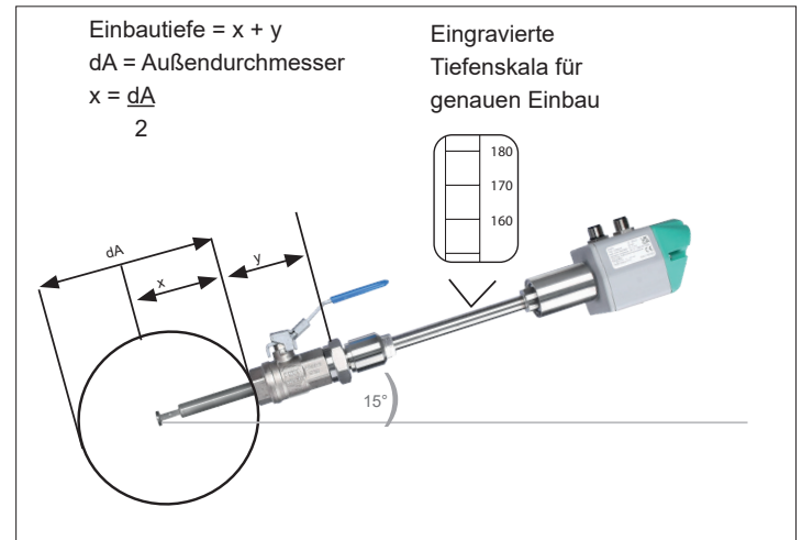
Empfohlene Einbaulage
