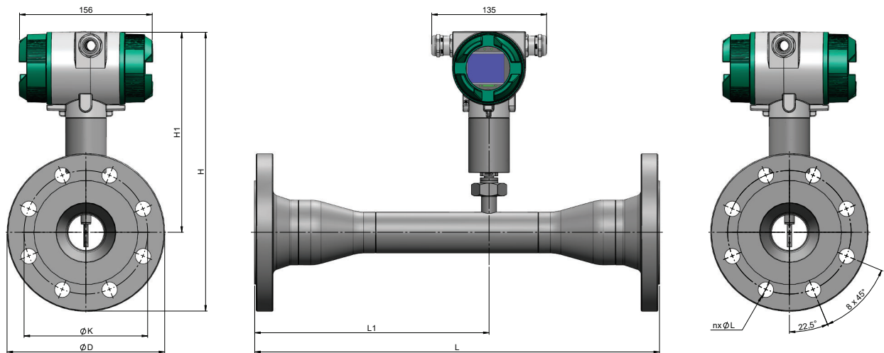
VD 570 - Sección de medición reducida con brida (Material stainless steel: 1.4404)
