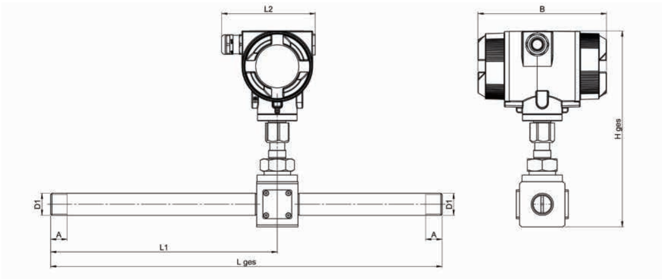
VU 570 - 带螺纹
